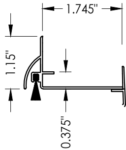
45 DOOR SWEEP
